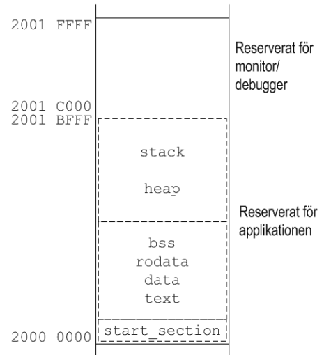
FIGUR 2: ANVÄNDNING AV RWM I MD407
