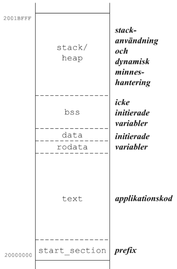
FIGUR 3: MINNESANVÄNDNING FÖR PROGRAM UNDER EXEKVERING
